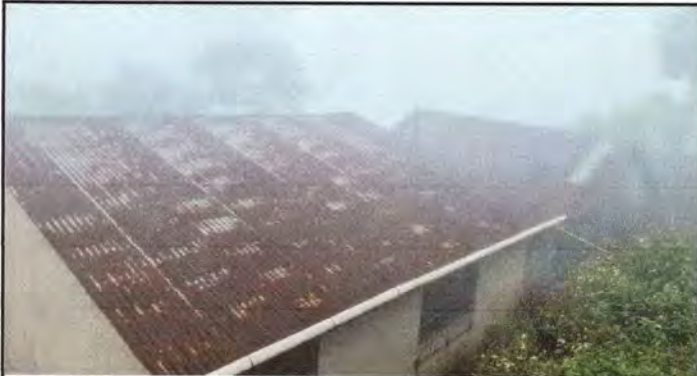
Foto 7: Sustrucción de lámina acanalada en mal estado por lámina troquelada para mejorar la calidad de los ambientes (aulas).
